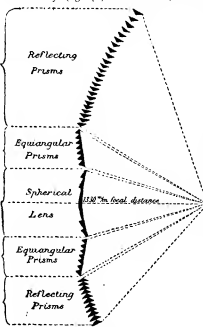
FIG. 40.—Sule Skerry Apparatus.
