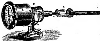
FIG. 4.—The Cherub Log.
