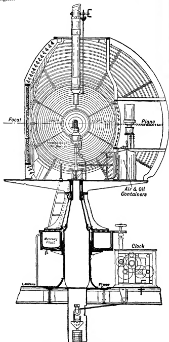
FIG. 42.—Cape Naturaliste Apparatus.
