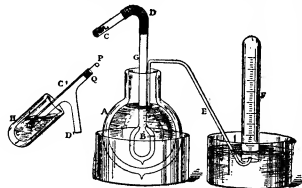
FIG. 13.—Calorimetric Apparatus.
