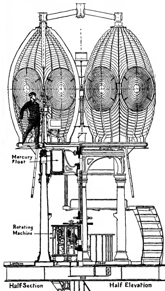
FIG. 43.—De Vierge Apparatus.
