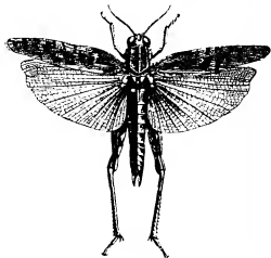
FIG. 3.— Caloptenus italicus .
