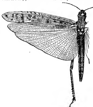
FIG. 2.— Acridium peregrinum .
